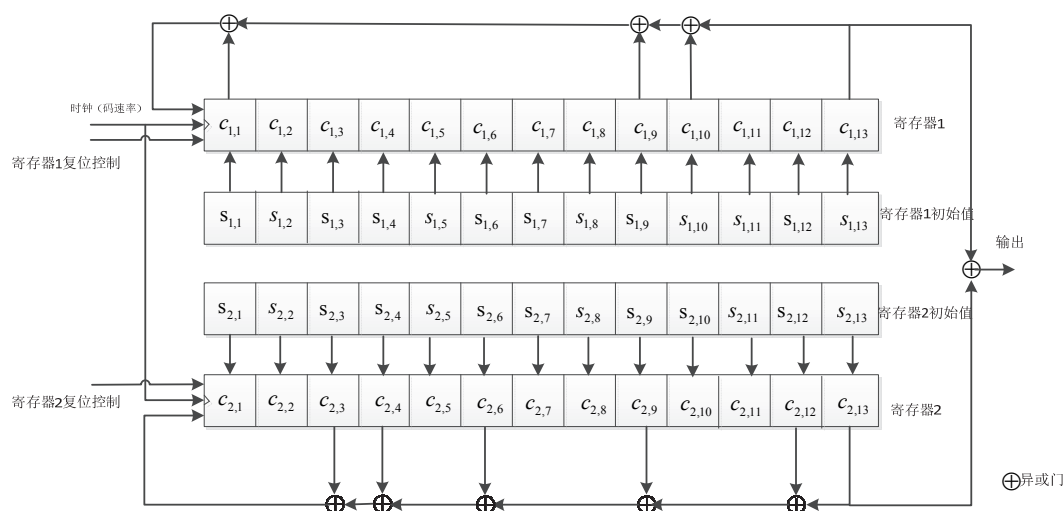
图 5-1 PPP-B2b I 支路测距码发生器
