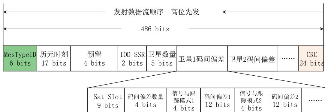
图 6-5 信息类型 3 格式编排
