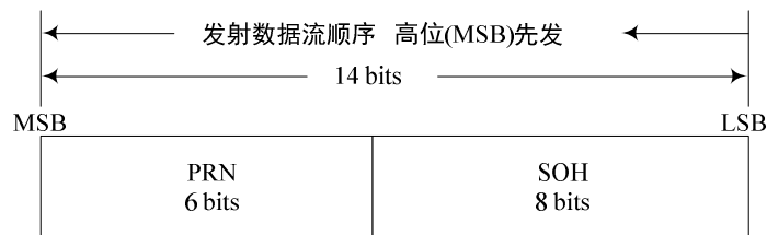
图 6-5 B-CNAV1 子帧 1 信息编排格式
