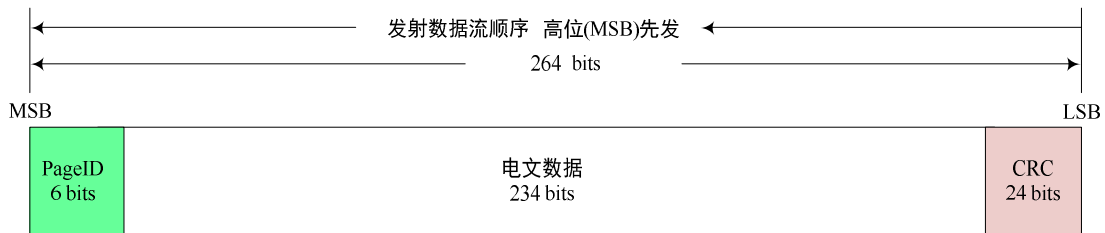
图 6-7 B-CNAV1 子帧 3 的帧结构
