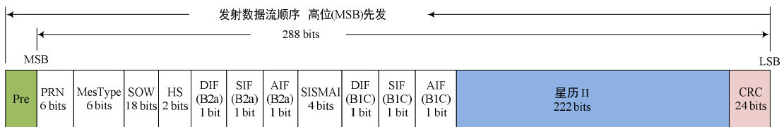
图 6-24 B-CNAV2 信息类型 11 编排格式
