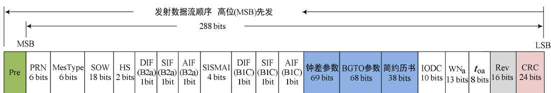
图 6-28 B-CNAV2 信息类型 33 编排格式
