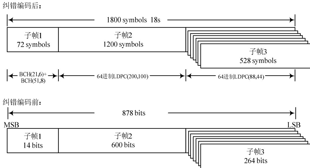
图 6-1 B-CNAV1 帧结构
