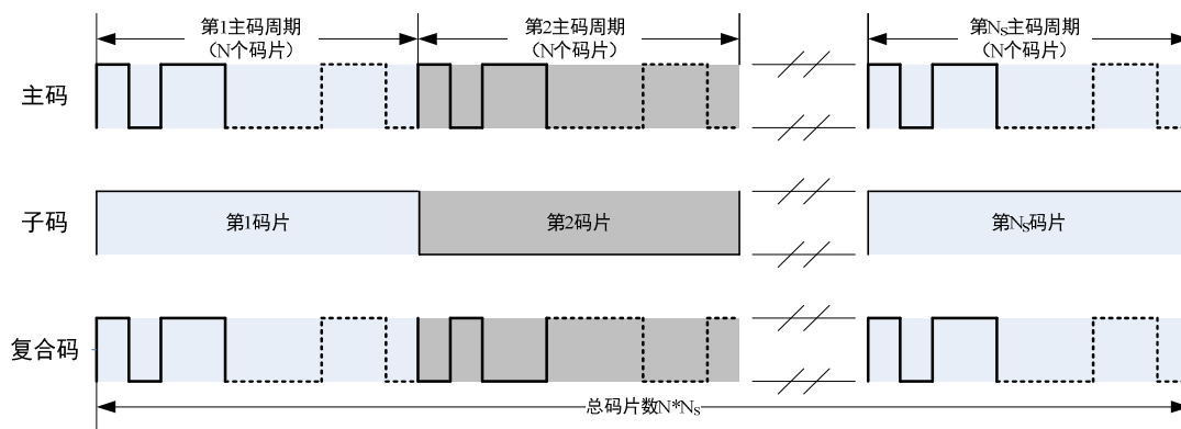
图 5-1 主码、子码时序关系示意图
