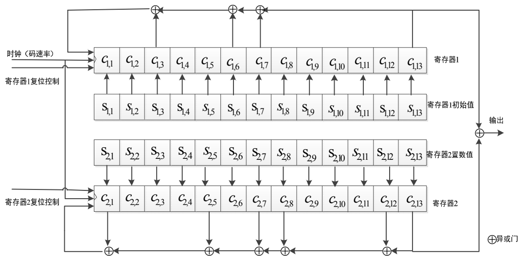
图 5-3 B2a 导频分量的主码发生器
