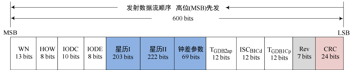
图 6-6 B-CNAV1 子帧 2 信息编排格式
