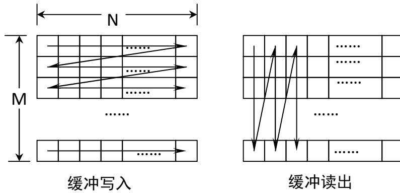
图 6-4 块交织过程示意图
