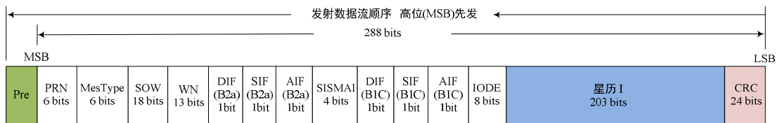
图 6-23 B-CNAV2 信息类型 10 编排格式
