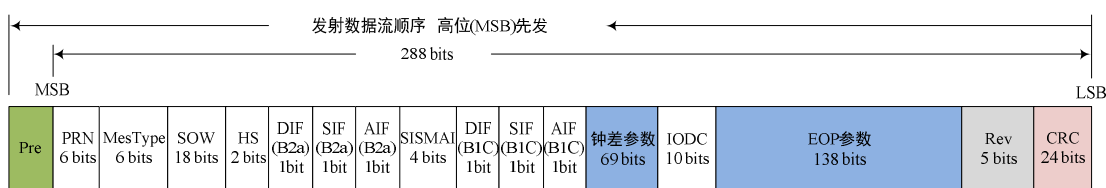
图 6-27 B-CNAV2 信息类型 32 编排格式
