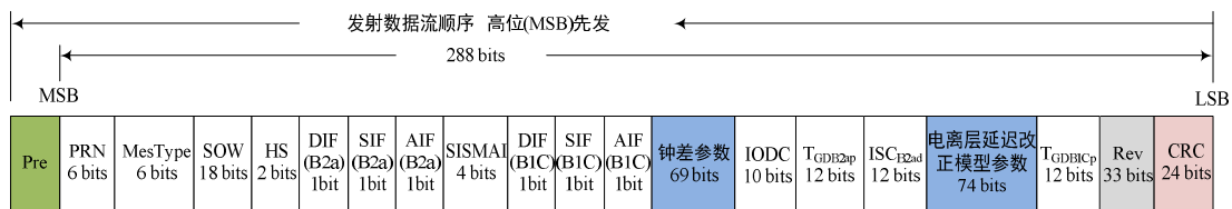
图 6-25 B-CNAV2 信息类型 30 编排格式
