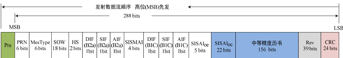
图 6-30 B-CNAV2 信息类型 40 编排格式
