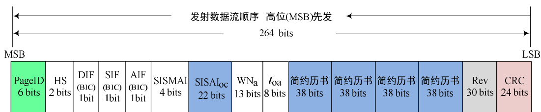
图 6-9 B-CNAV1 子帧 3 页面类型 2 信息编排格式
