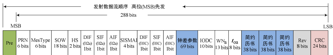
图 6-26 B-CNAV2 信息类型 31 编排格式
