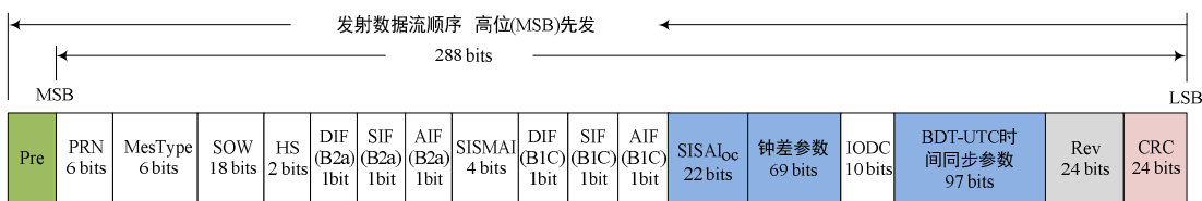
图 6-29 B-CNAV2 信息类型 34 编排格式
