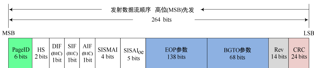
图 6-10 B-CNAV1 子帧 3 页面类型 3 信息编排格式
