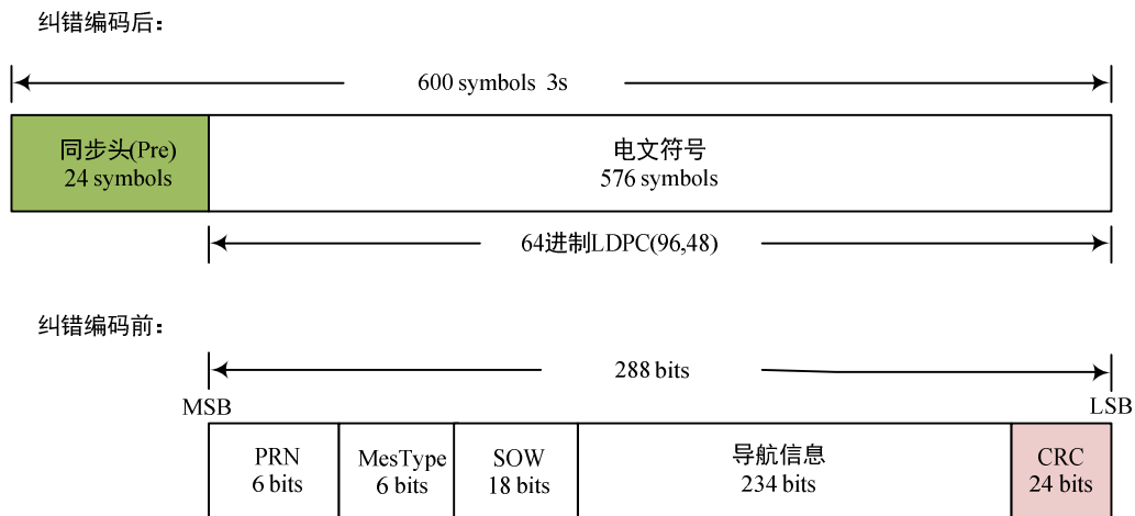
图 6-22 B-CNAV2 帧结构
