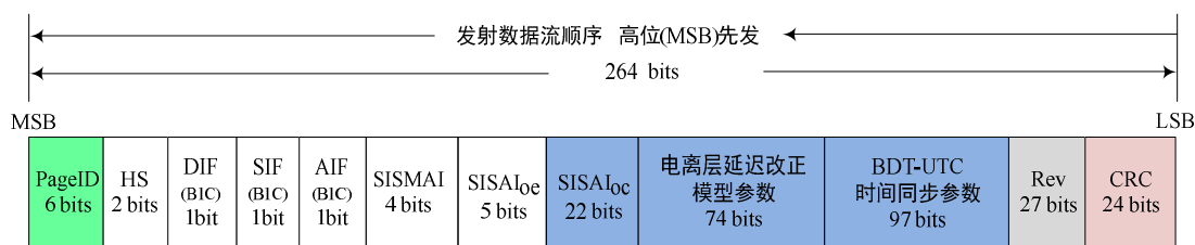
图 6-8 B-CNAV1 子帧 3 页面类型 1 信息编排格式
