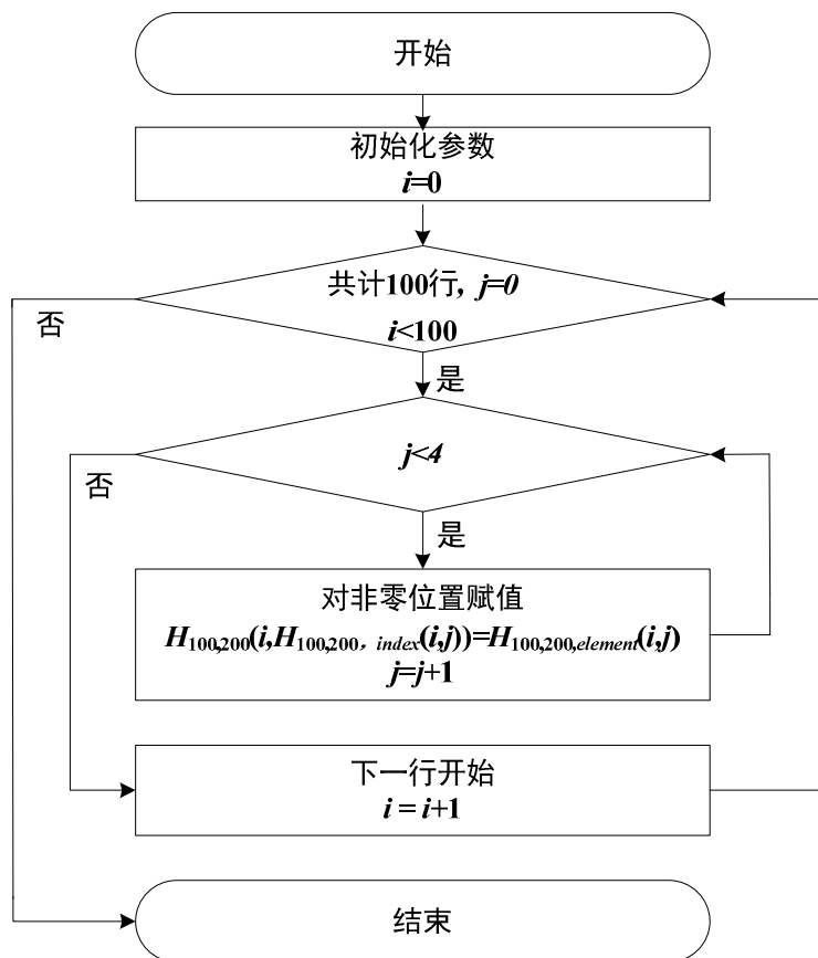
图 6-3 H 100,200 读取流程图
