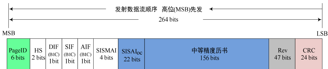
图 6-11 B-CNAV1 子帧 3 页面类型 4 信息编排格式
