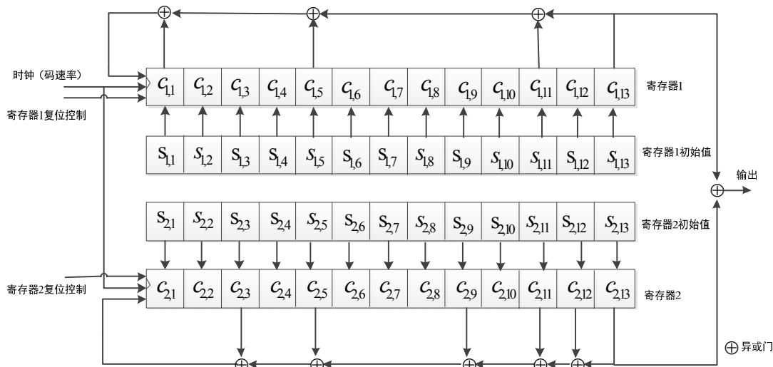
图 5-2 B2a 数据分量的主码发生器
